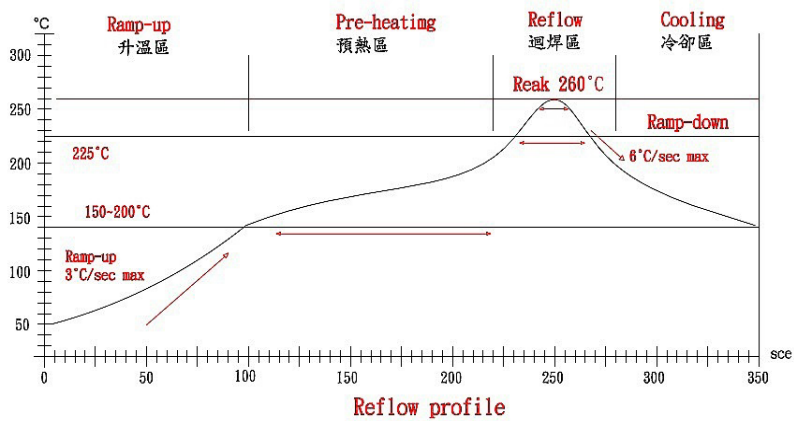
Lead-Free(LF)標準溫度分析範圍
