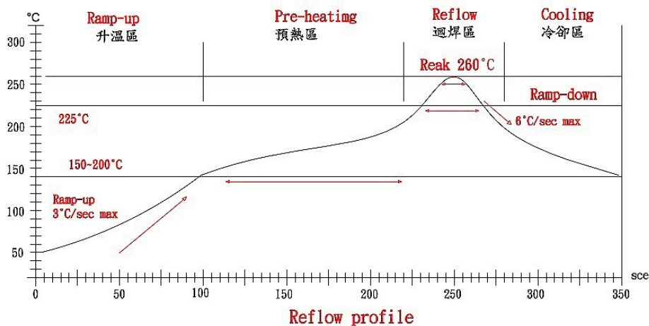
Lead-Free(LF)標準溫度分析範圍
